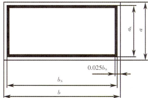
图 A. 5 附加提示标识的基本形式
